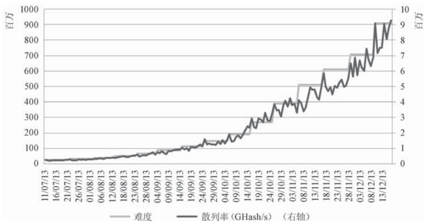
图3 挖矿难度
